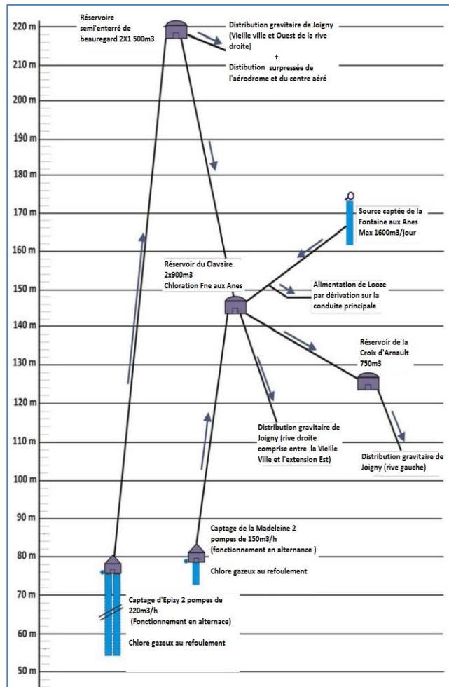
Schéma simplifié du système de production distribution d'eau
